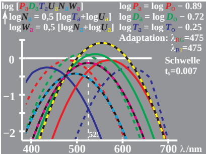
WG770-1, Änderung von PDT (LMS) beim Farbsehen; Adaptation
