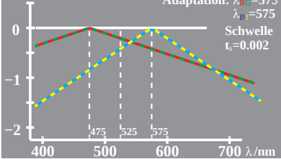
WG741-7, Änderung von PDT (LMS) beim Farbsehen; Adaptation
