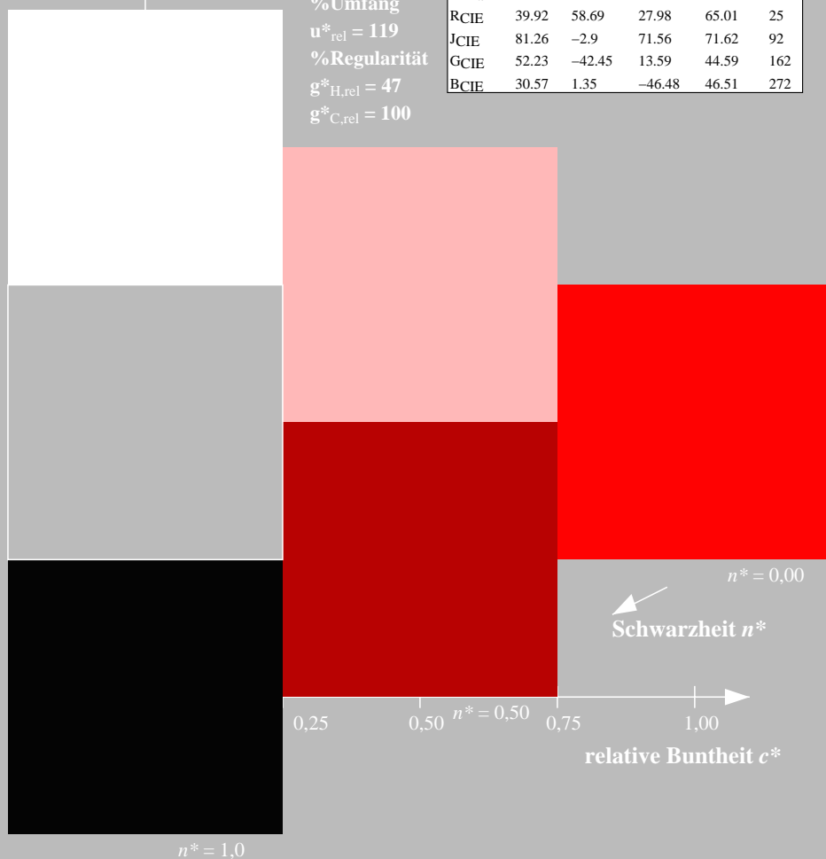
TG070-7, 3 stufige Reihen für konstanten CIELAB Buntton 24/360 = 0.067 (links)
