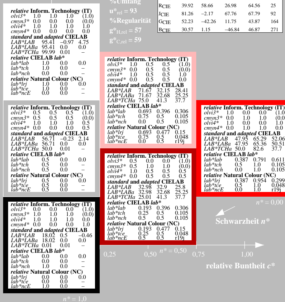
3 stufige Reihen für konstanten CIELAB Buntton 38/360 = 0.105 (rechts)
