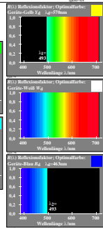
Wellenlängenbereiche für CIE-Normlichtart D65
