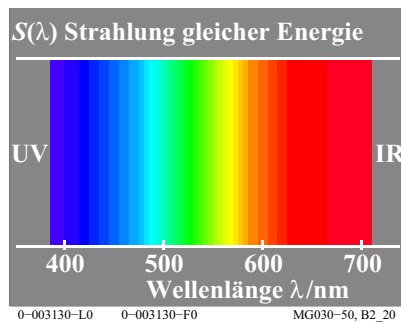
Bild 20: Sichtbarer Spektralbereich
