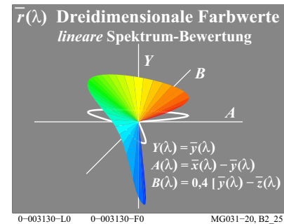
Bild 23: Dreidimensionale Farbwerte
