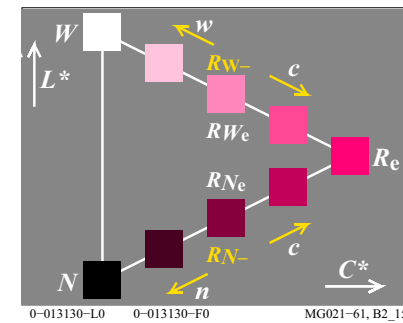
Bild 16: Maximale Buntheit
