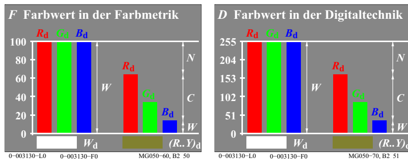
Bild 37: Trichromatische Farbwerte RGB_d in Farbmeterik und Digitaltechnik
