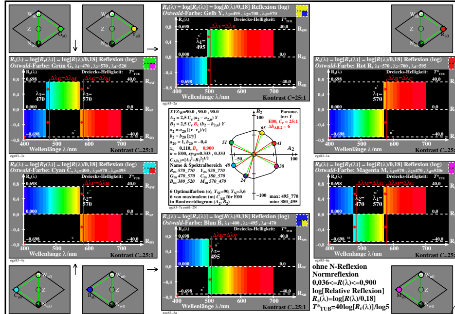
TUB-Prüfvorlage egz8; Wellenlängenbereiche von 6 Ostwald-Farben und Weiß W, +/- Signale Reflexionen R(\lambda) , R_r(\lambda) = R(\lambda) / 0,18 und R_s(\lambda) = \log[R_r(\lambda)] , Bunttonschwelle \Delta h_{A_2B_2} = 6 , C = 25:1
