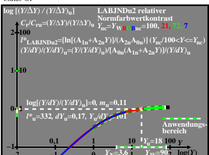
CGH20-8A
