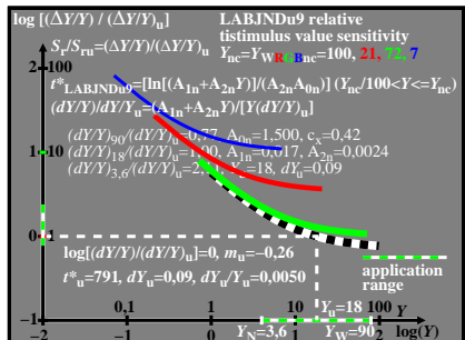
CEE90-6A
