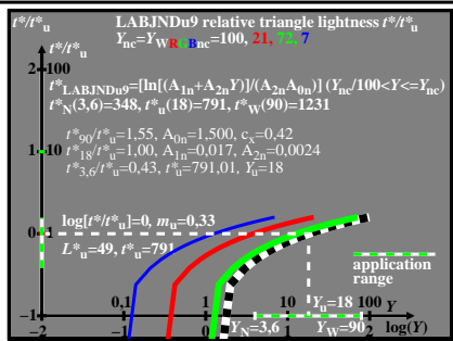
CEE90-2A
