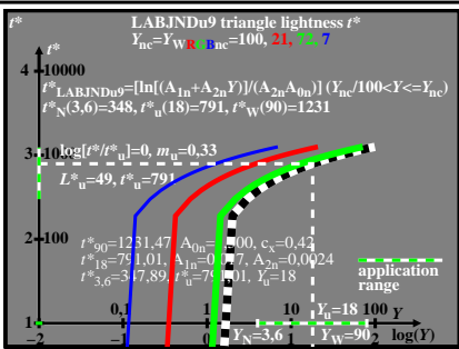
CEE90-1A
