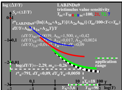
CEE90-5A
