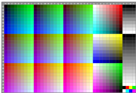
AEA60-7N, File: http://farbe.li.tu-berlin.de/AEA6/AEA60-7N.EPS , 1MR, gamma \gamma=0.849 , C_{Y16}
